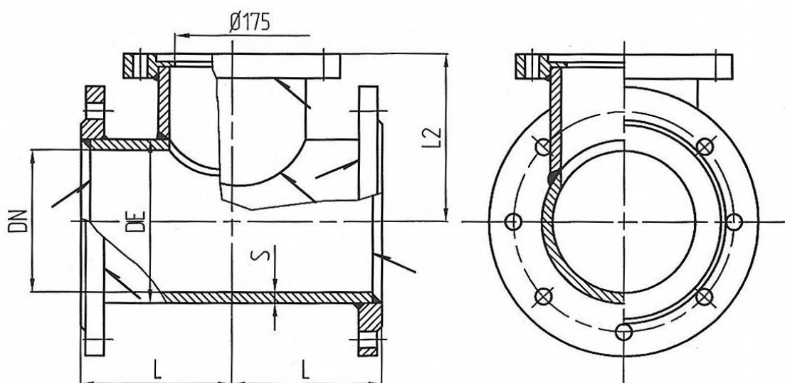
Пожарная подставка раструбная свыше DN150 мм
