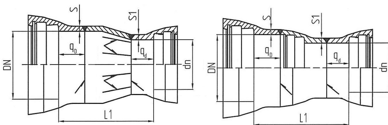
Рисунок 12.21 - Переход раструбный (ХР)
