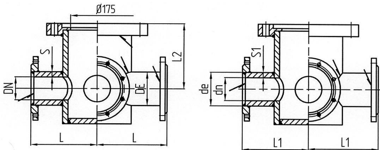
Крест фланцевый с пожарной подставкой DN100-150 мм
