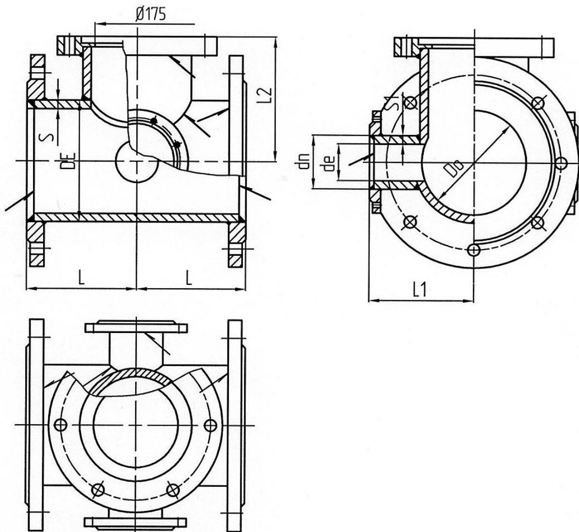
Крест фланцевый с пожарной подставкой свыше DN150 мм
