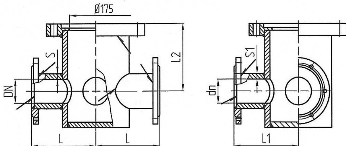
Тройник фланцевый с пожарной подставкой DN100-150 мм
