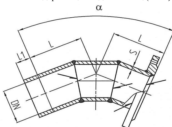
Отвод фланец - гладкий конец (ОФГ)
