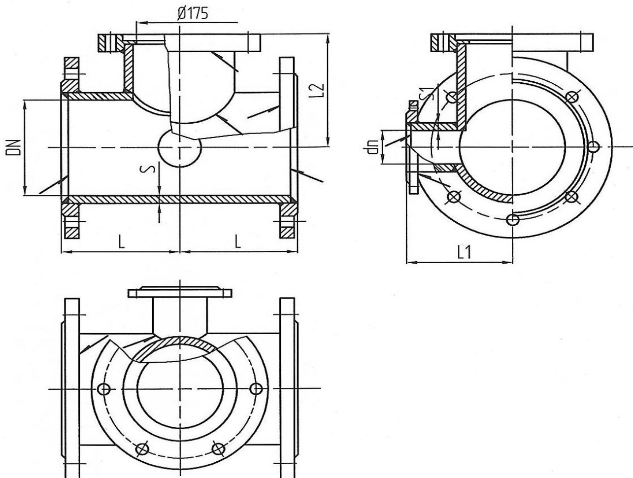
Тройник фланцевый с пожарной подставкой DN100-150 мм
