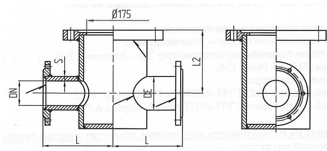
Пожарная подставка фланцевая DN100-150 мм
