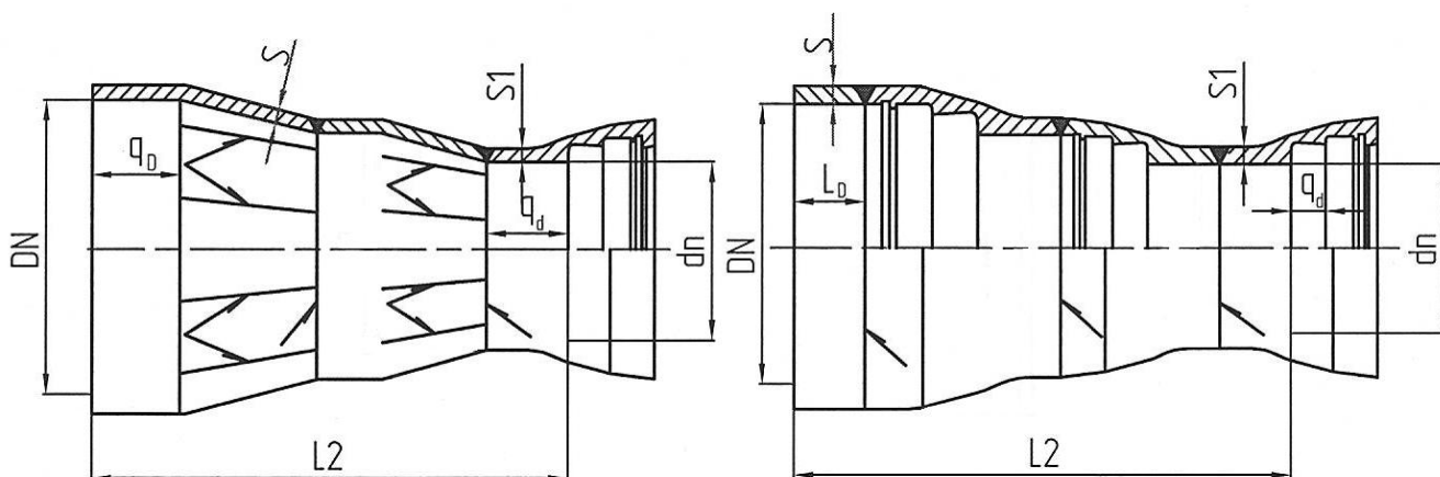
Рисунок 12.22 - Переход раструб – гладкий конец (ХРГ)
