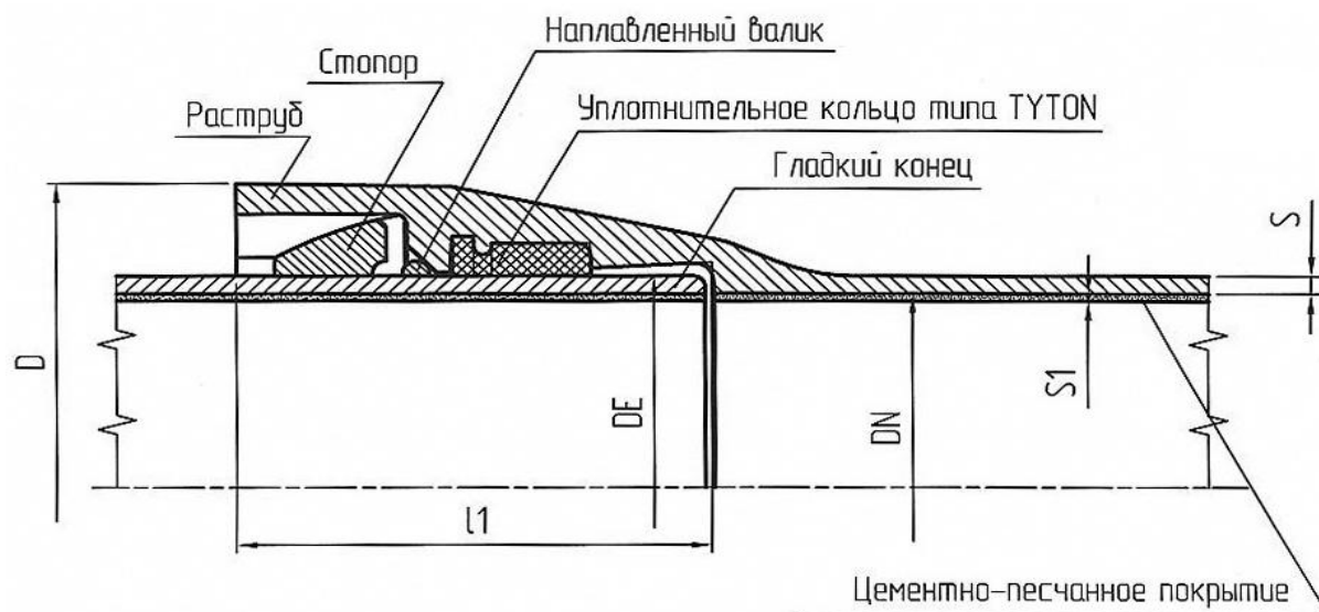
Рисунок А.2 – Раструбно-замковое соединение «RJ»: а) – с уплотнительным резиновым кольцом типа «BPC»; б) - с уплотнительным резиновым кольцом типа «TYTON».
