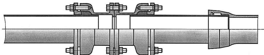
Рисунок. Ремонт трубопровода при помощи патрубка фланец - раструб компенсационный ПФРК.
