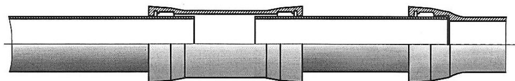
Рисунок. Ремонт трубопровода при помощи подвижной муфты МН.
