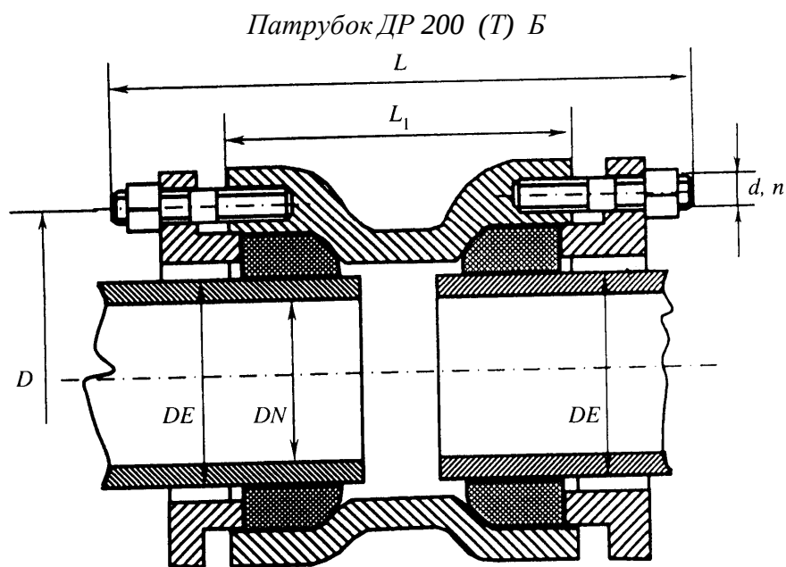
Рисунок Б.21 — Двойной раструб компенсационный
