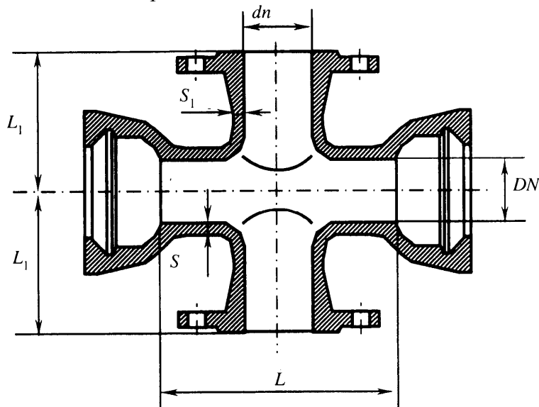
Рисунок Б.27 — Крест раструб-фланец
