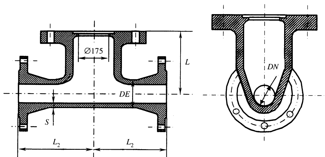
Рисунок Б.35 — Пожарная подставка фланцевая
