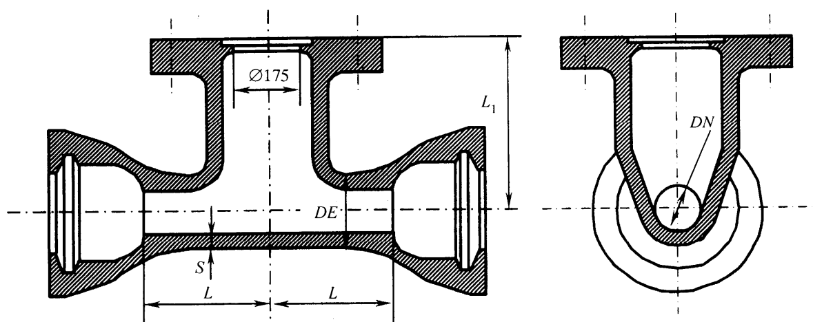
Деталь построения фланца под пожарный кран
