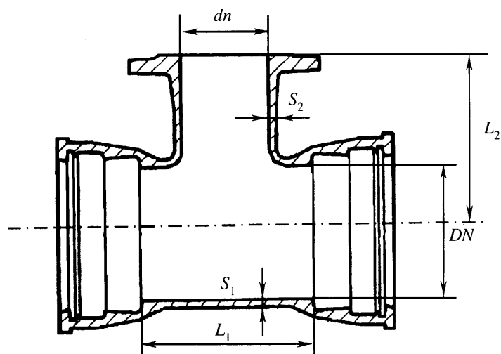
Рисунок Б.4 — Тройник раструб-фланец
