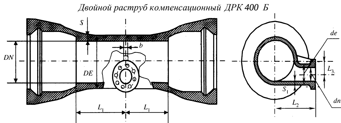
Рисунок Б.22 — Выпуск раструбный
