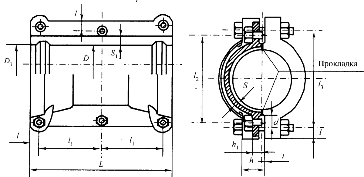
Рисунок Б.32 — Муфта свертная
