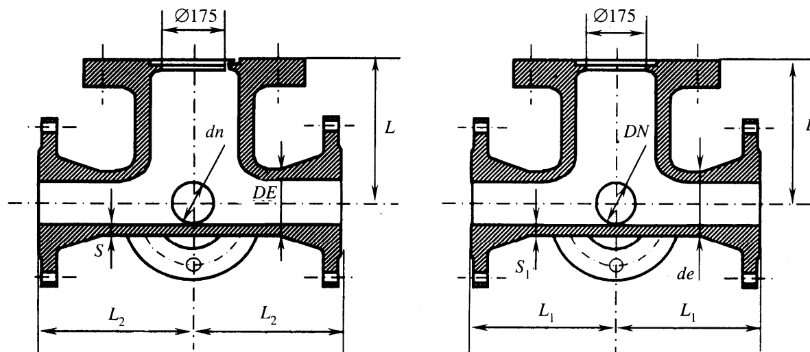
Рисунок Б.31 — Крест фланцевый с пожарной подставкой
