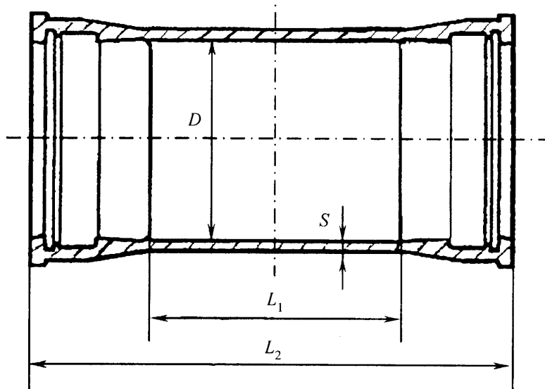
Рисунок Б.33 — Муфта надвижная
