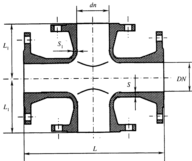
Рисунок Б.29 — Крест фланцевый
