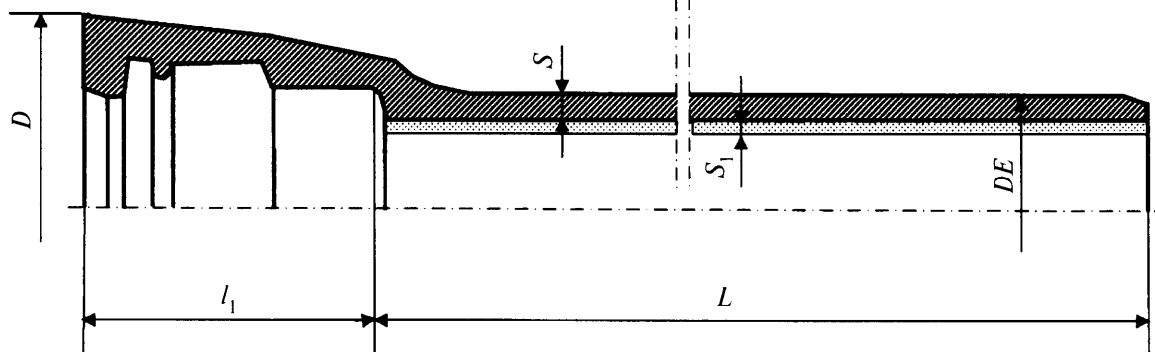
Рисунок А.1 — Труба раструбная под соединение «TYTON»
