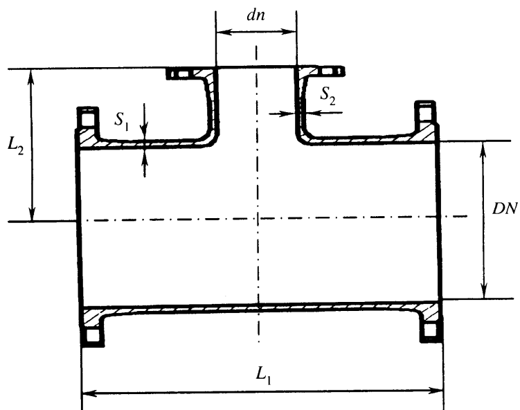
Рисунок Б.6 — Тройник фланцевый
