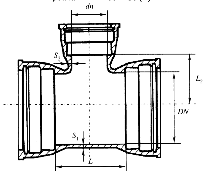
Рисунок Б.5 — Тройник раструбный
