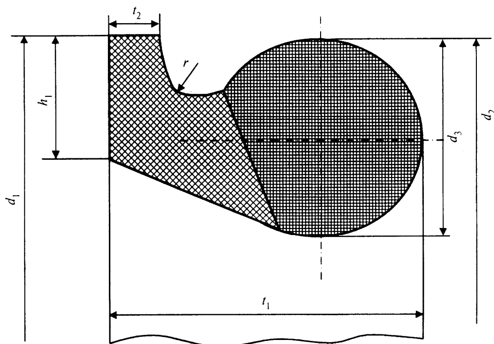
Рисунок А.7 — Уплотнительное резиновое кольцо под соединение «TYTON»
