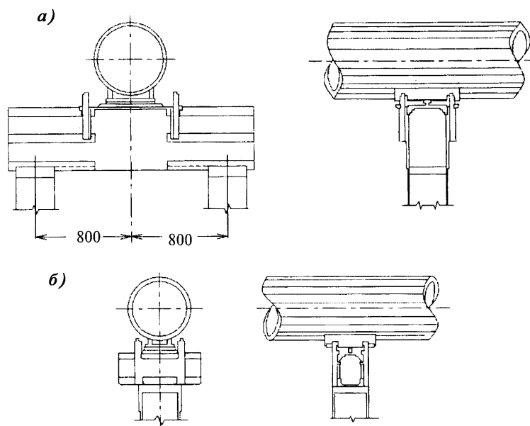
Рисунок 6.5 — Опорные железобетонные башмаки для труб диаметрами 400—500 мм под одну стойку (а), под две стойки (б)
