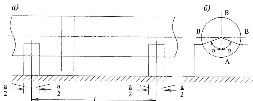
Рисунок 6.2 — Трубопровод на отдельных опорах
