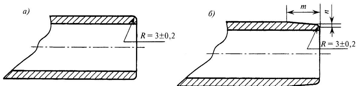
Рисунок А.5 — Торцы гладкого конца трубы
