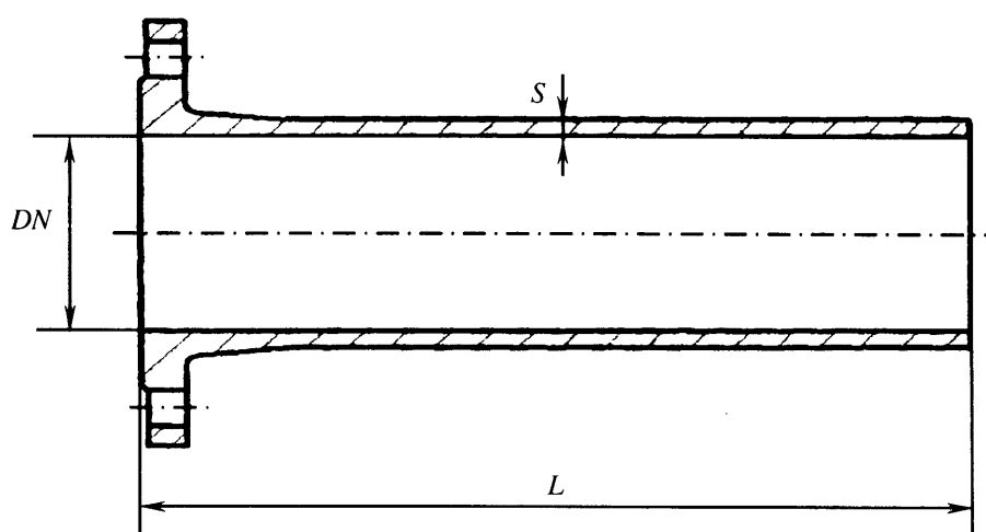
Рисунок Б.19 — Патрубок фланец — гладкий конец
