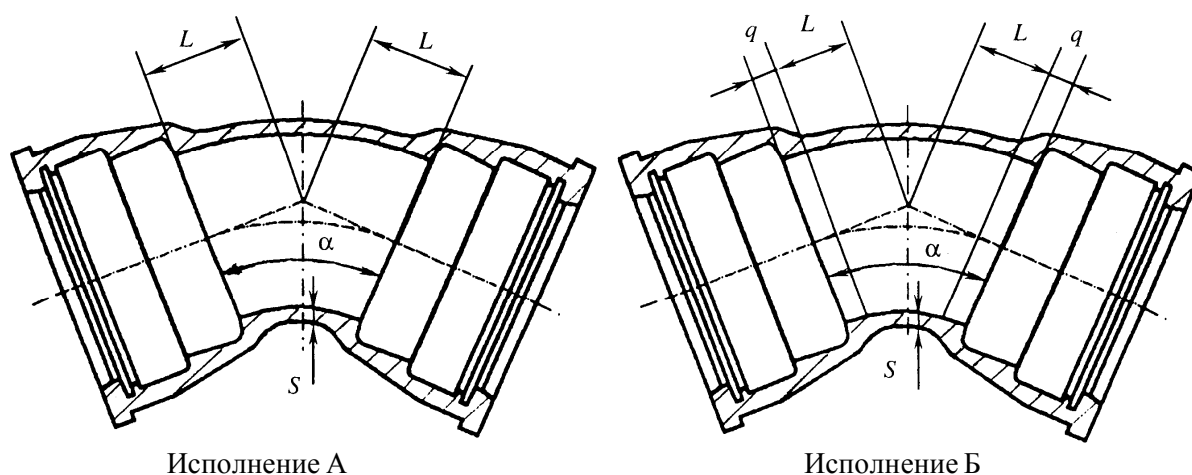
Рисунок Б.11 — Отвод раструбный
