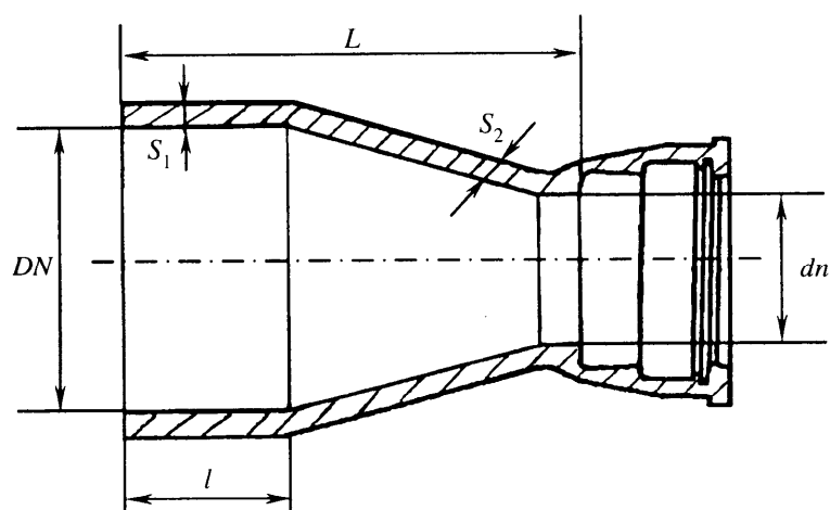
Рисунок Б.13 — Переходраструб — гладкий конец
