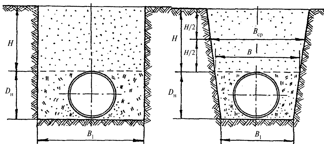
Рисунок 5.5 — Схемы укладки подземного трубопровода
