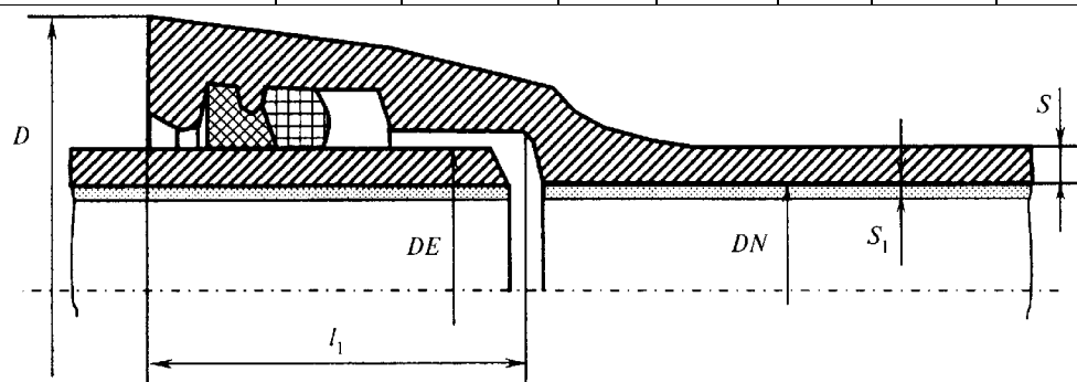
Рисунок Б.2 — Раструбное соединение типа «TYTON»
