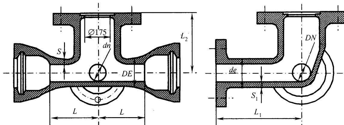
Рисунок Б.25 — Тройник раструб-фланец с пожарной подставкой
