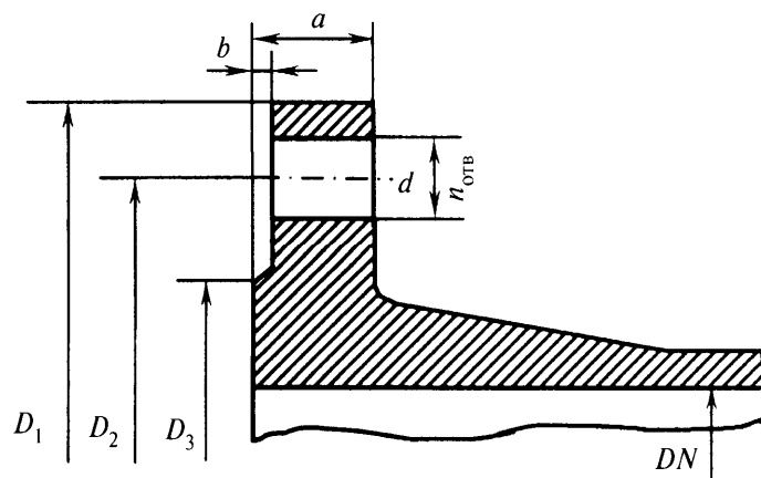
Рисунок Б.3 — Фланец
