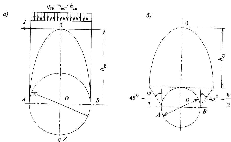
Рисунок 7.2 — Давление грунта на подземную трубу при образовании свода естественного равновесия
