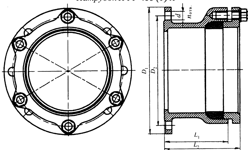
Рисунок Б.18 — Патрубок фланец — раструб компенсационный
