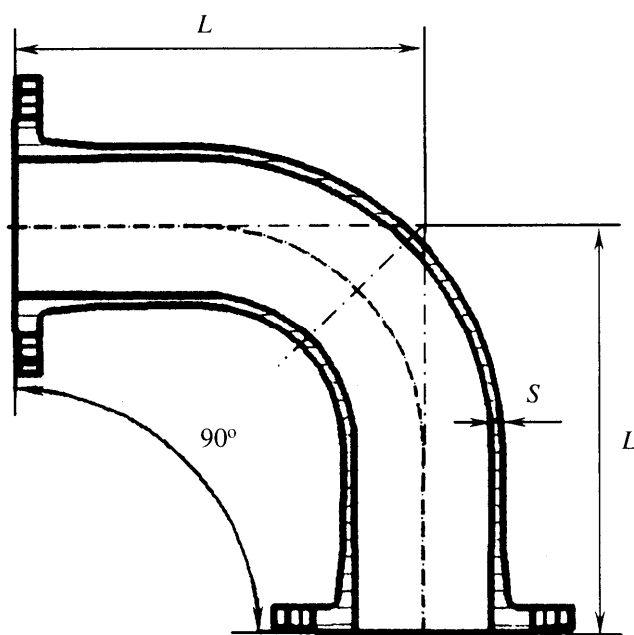
Рисунок Б.8 — Колено фланцевое
