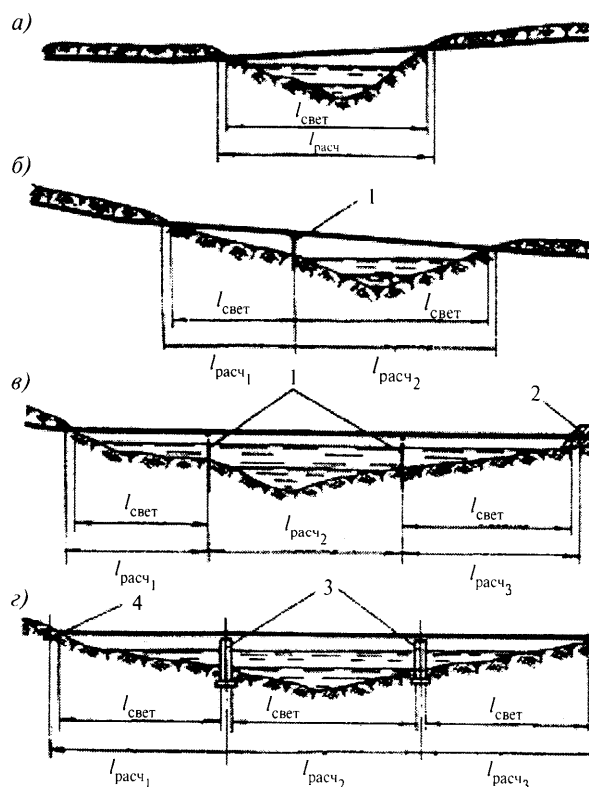
а — однопролетный наклонный; б — двухпролетный наклонный с разной величиной пролетов; в — трехпролетный со свайными опорами; г — трехпролетный с массивными промежуточными опорами и плитными опорами по концам; 1 — свайная опора; 2 — насыпь; 3 — массивные опоры; 4 — железобетонная плита
