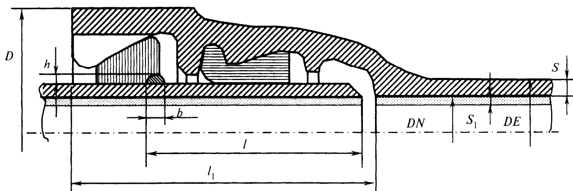
Рисунок Б.1 — Раструбное соединение типа «RJ»
