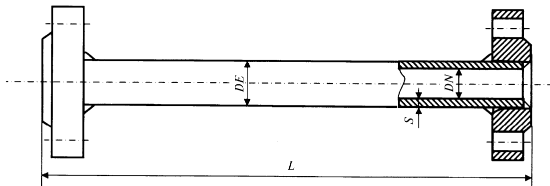
Рисунок А.3 — Труба с приваренными фланцами
