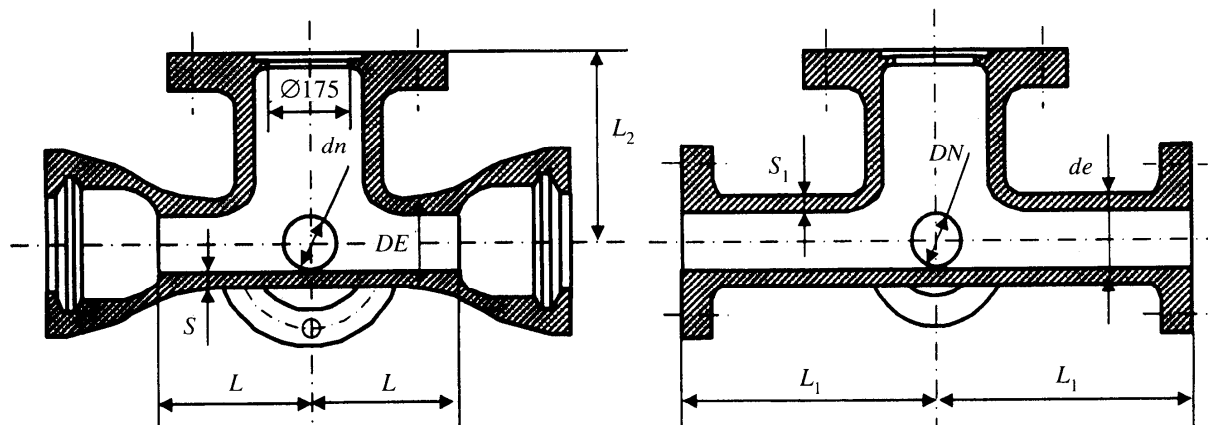
Рисунок Б.30 — Крест раструб-фланец с пожарной подставкой
