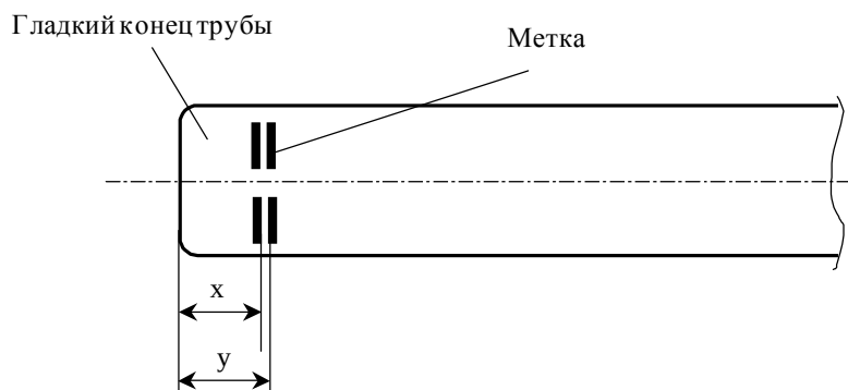
Рисунок 5.8 — Нанесение меток. Метка у равна глубине раструба, а x = y - 10 мм, для всех диаметров труб
