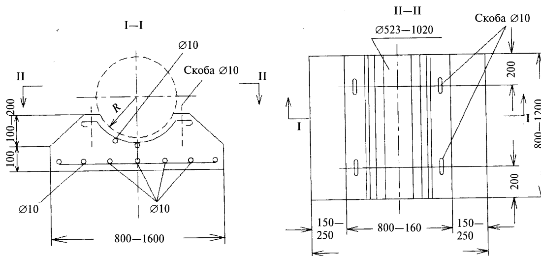
Рисунок 6.4 — Плитная опора с ложем для укладки трубопровода
