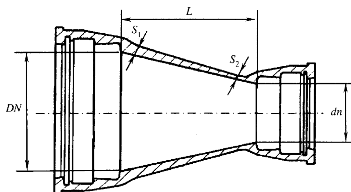
Рисунок Б.16 — Переходраструбный
