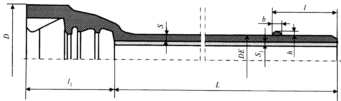
Рисунок А.2 — Труба раструбная под соединение «RJ»
