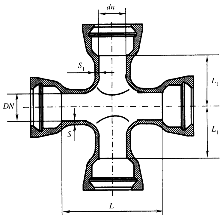
Рисунок Б.28 — Крест раструбный
