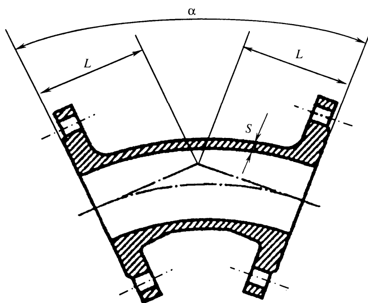
Рисунок Б.12 — Отвод фланцевый
