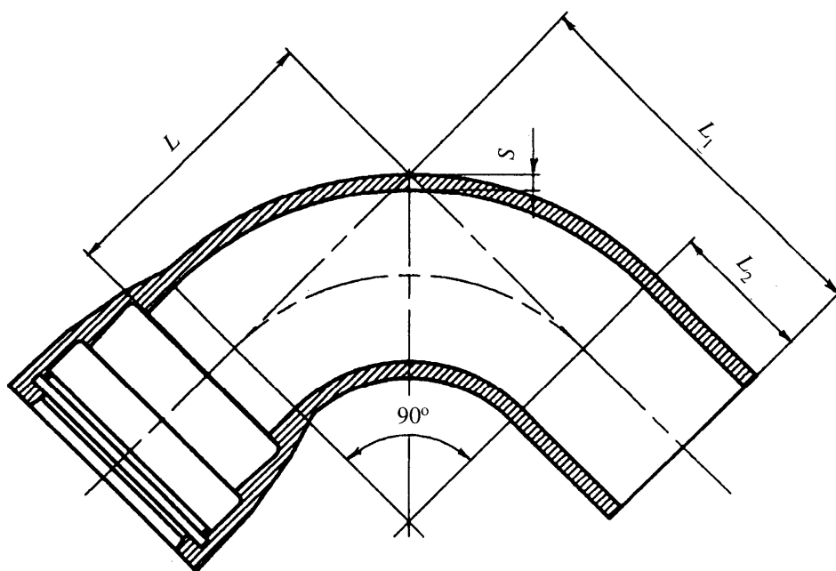
Рисунок Б.7 — Колено раструб-гладкий конец
