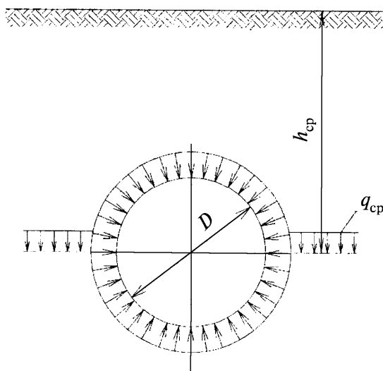
Рисунок 7.1 — Среднее давление грунта на подземный трубопровод
