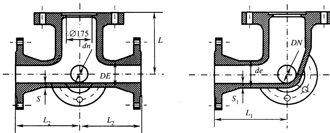
Рисунок Б.26 — Тройник фланцевый с пожарной подставкой
