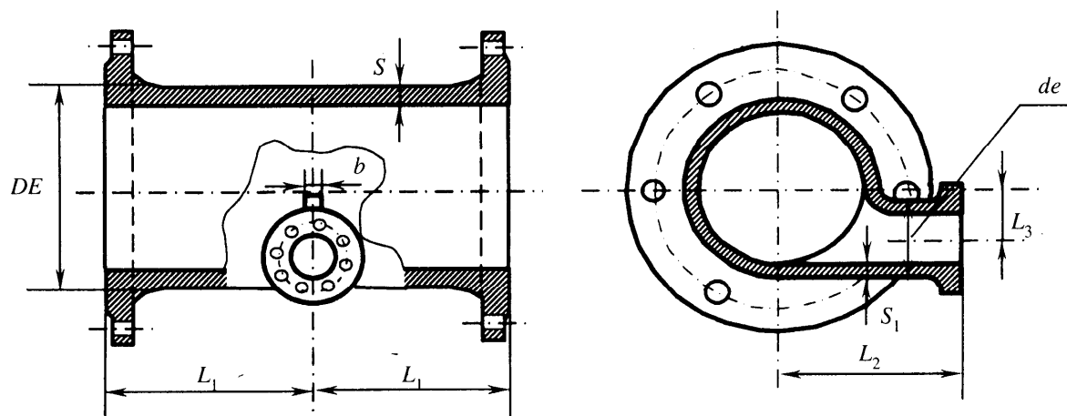
Рисунок Б.23 — Выпуск фланцевый
