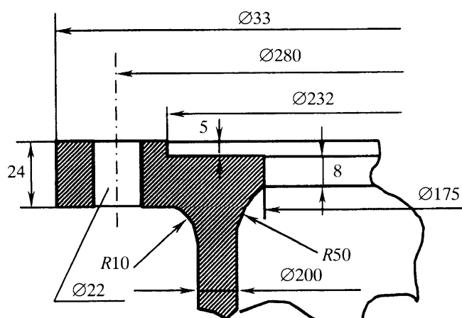
Рисунок Б.24 — Пожарная подставка раструбная
