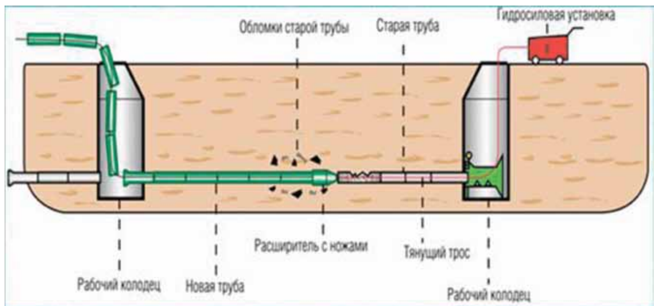
Рис. 11. Подземная прокладка с разрушением старого трубопровода
